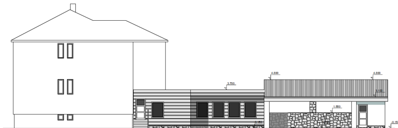
POHLED JIHOVÝCHODNÍ
